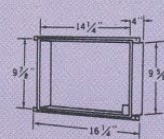
Model 2401-A and 2402-A Rough-in Box
